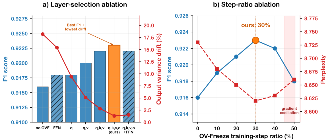
图 5: 正交泛化冻结策略 (OV-Freeze) 消融。a) 敏感层方差漂移的对齐演进特征: 全量激活 q, k, v, o 注意力算子能最大化收紧统计偏差; b) 动态激活时间步比例的收敛: 30% 的相对步长在梯度平稳度与保真度之间达到了帕累托最优。
